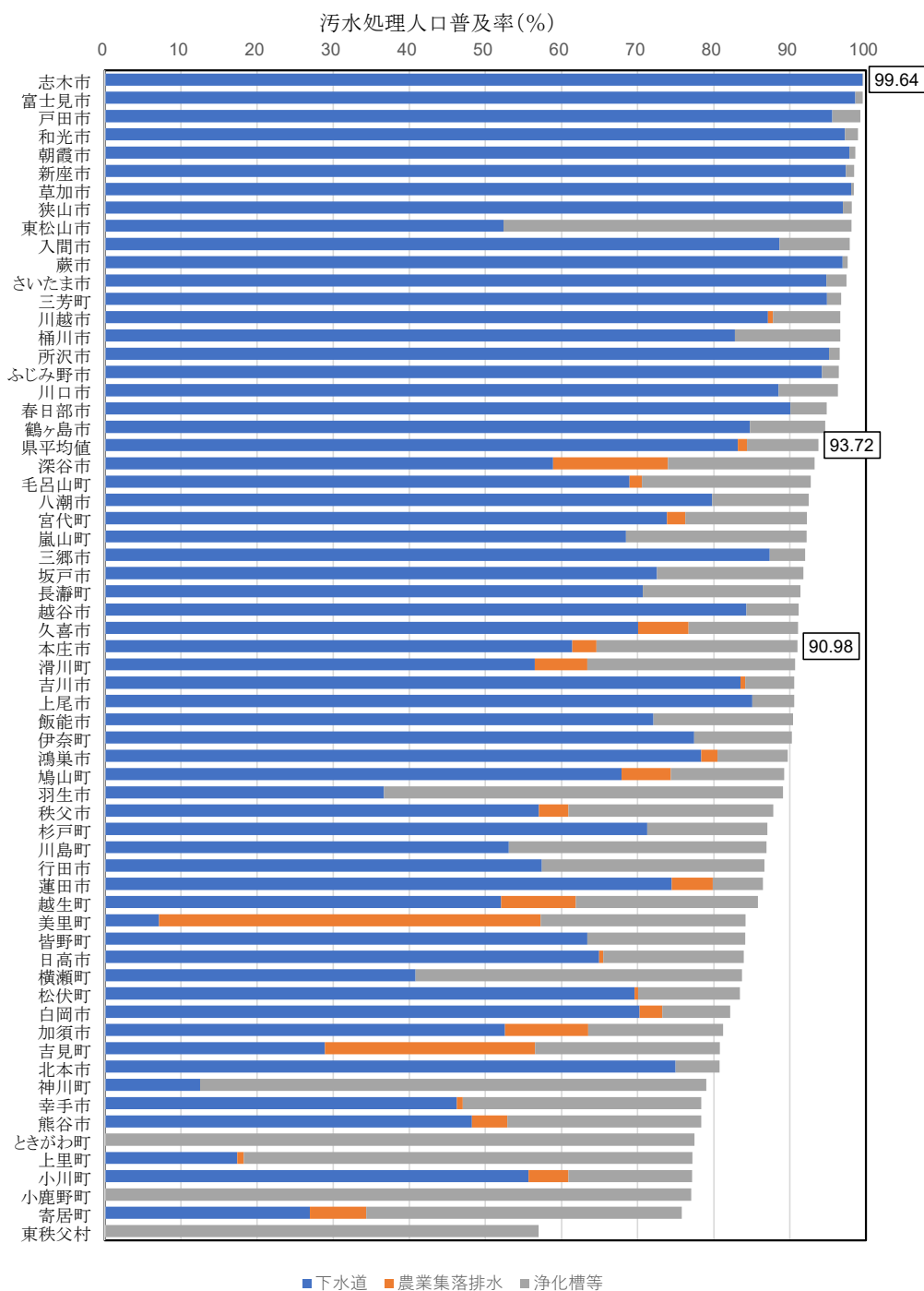
図 2-4-3 市町村別汚水処理人口普及率(令和 3(2021)年度)
