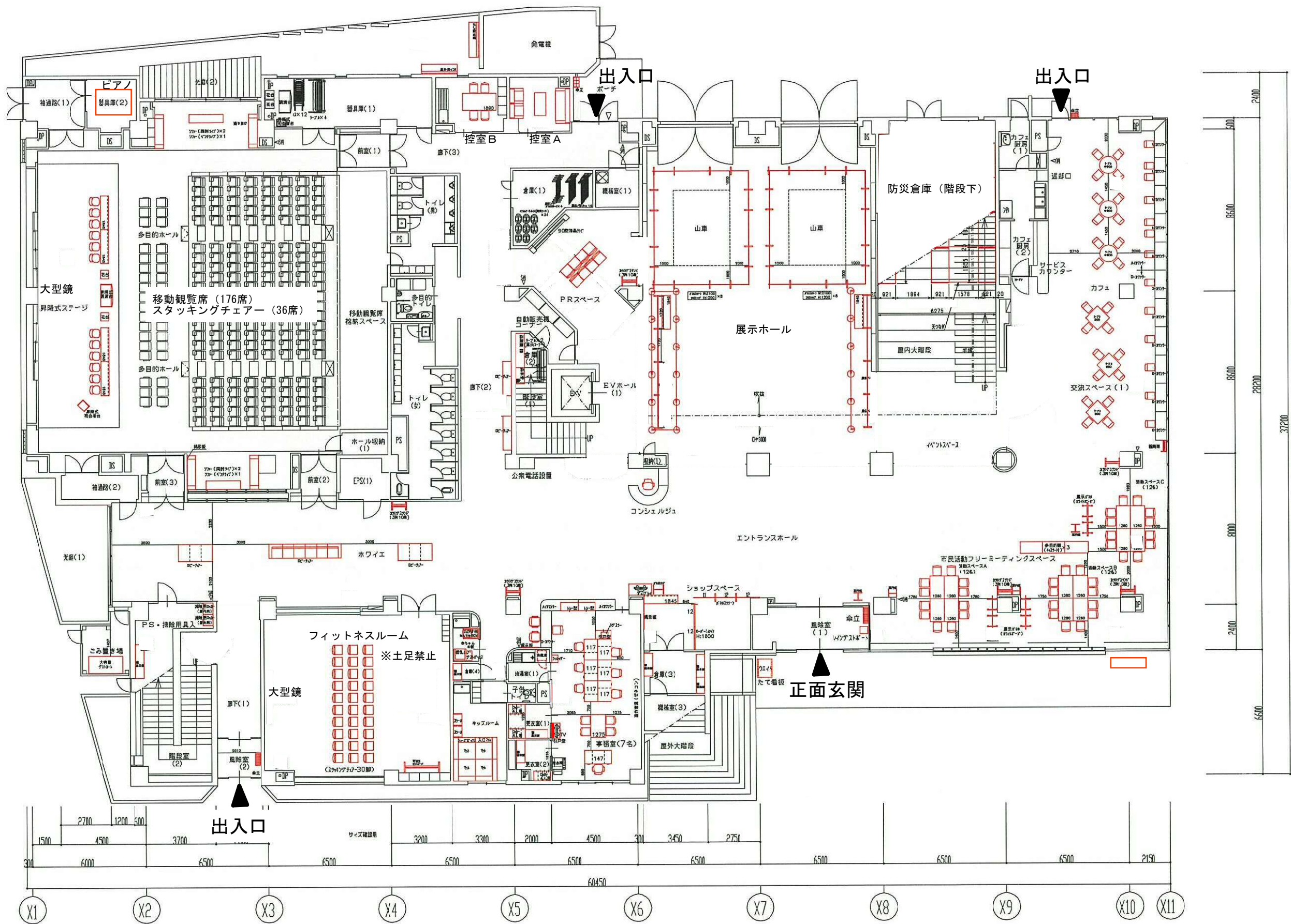
本庄市市民活動交流センター（はにぽんプラザ）1階備品配置図【予定】
