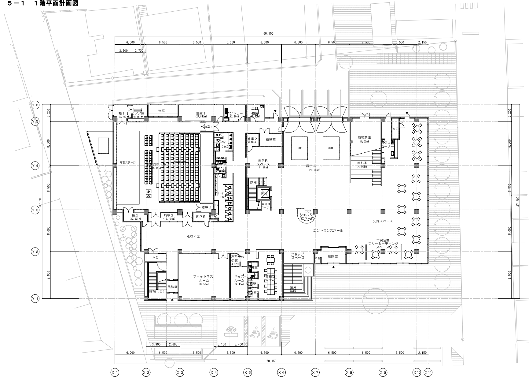
1階平面計画図 / 1,890㎡
