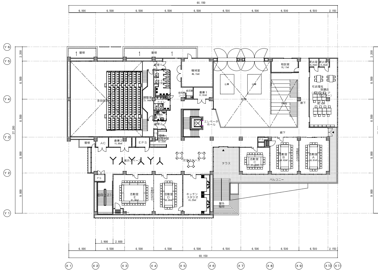
2階平面計画図 / 1,215㎡ Scale: 1/300
