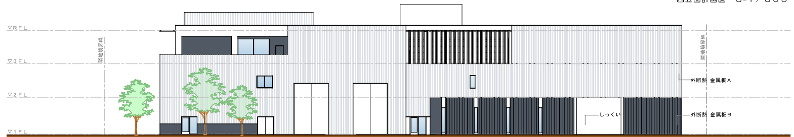
北立面計画図 S=1/300
