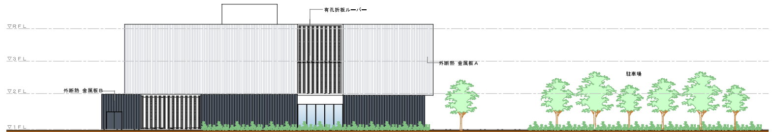
西立面計画図 S=1/300
