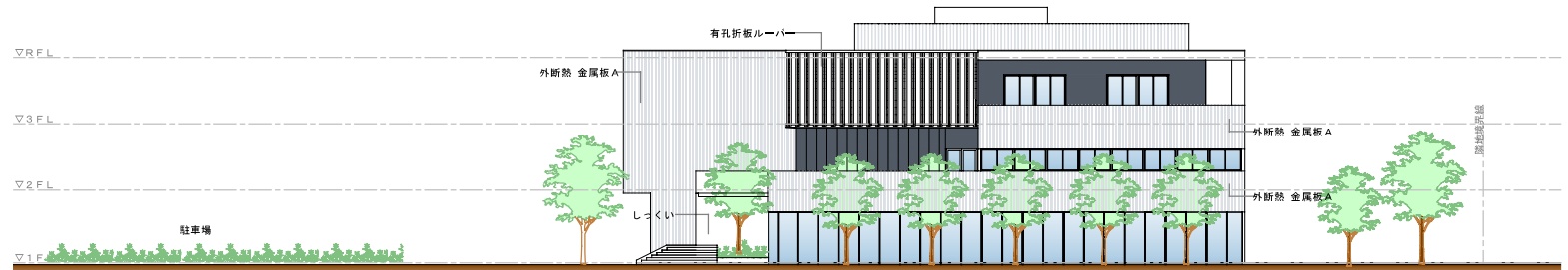
東立面計画図 S=1/300
