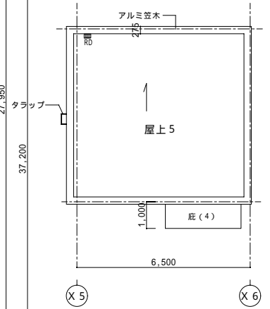
P H R階 平面図 S = 1/100
