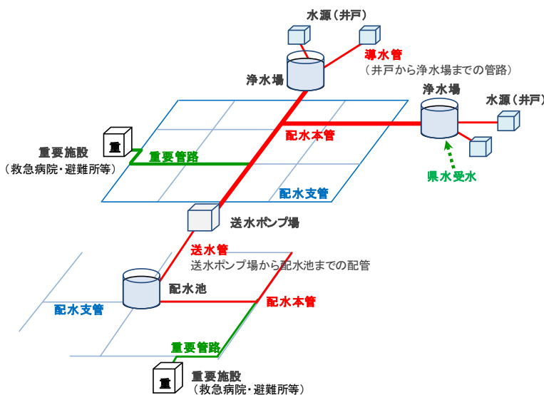
図5-2-3 管路の模式図
