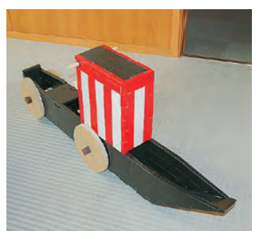
陸船車模型
